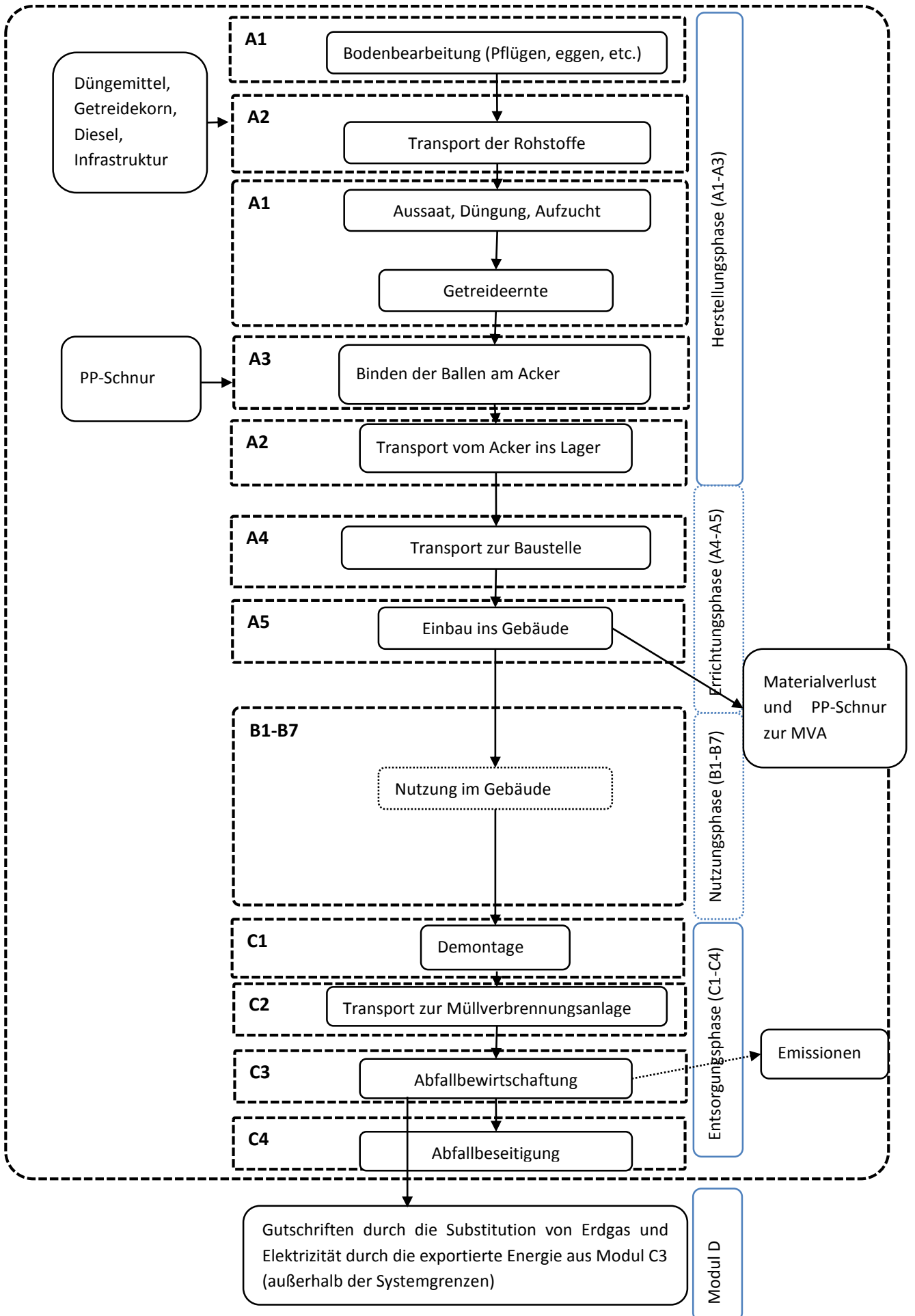
Abbildung 1: Flussdiagramm der Produktlebensphasen der Baustrohballen
