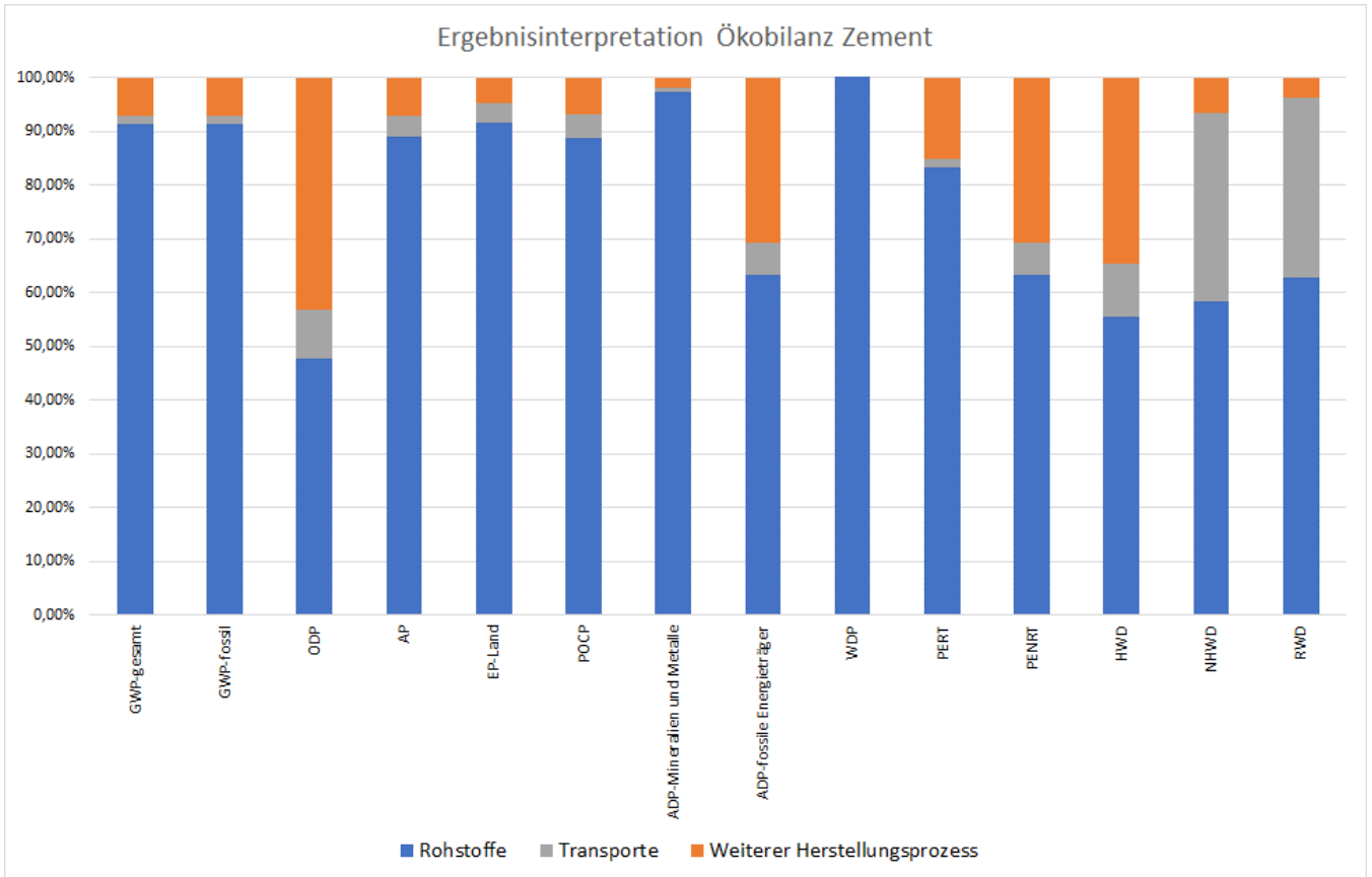
Abbildung 4: Dominanzanalyse Zementherstellung CEM II/C-M (S-LL) 42,5 N
