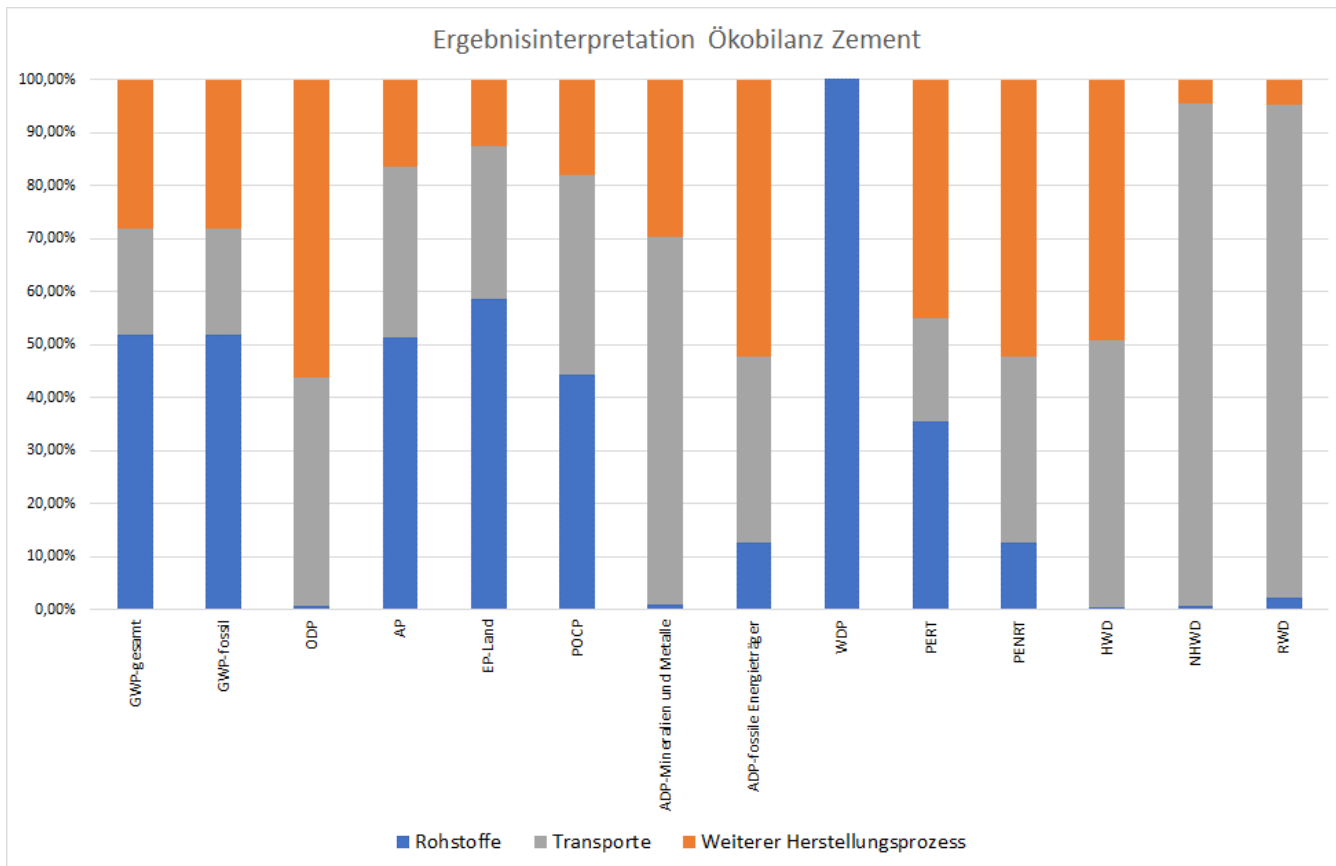
Abbildung 6: Dominanzanalyse Herstellung AHWZ-GS
