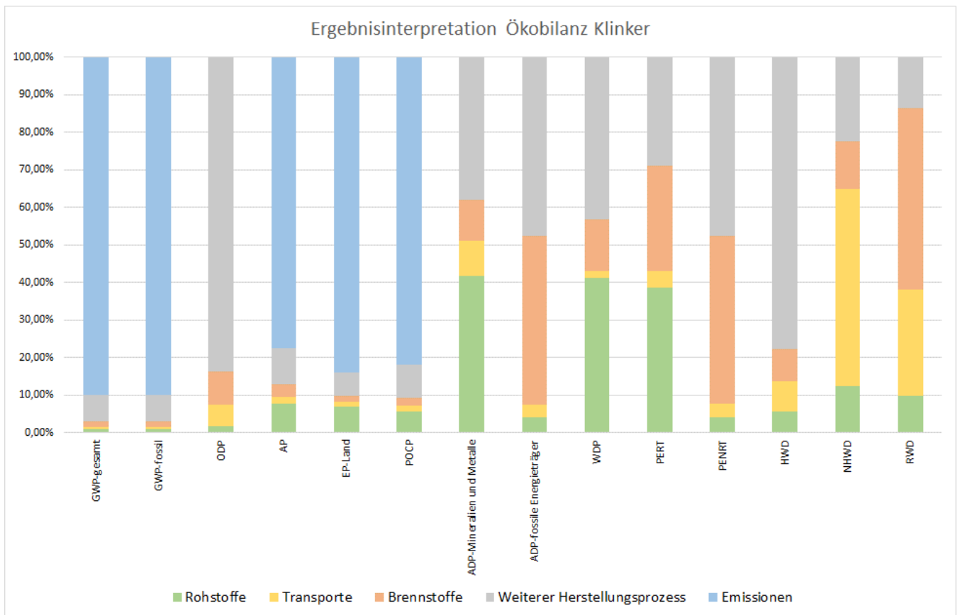
Abbildung 3: Dominanzanalyse Klinkerherstellung Baumit GmbH
