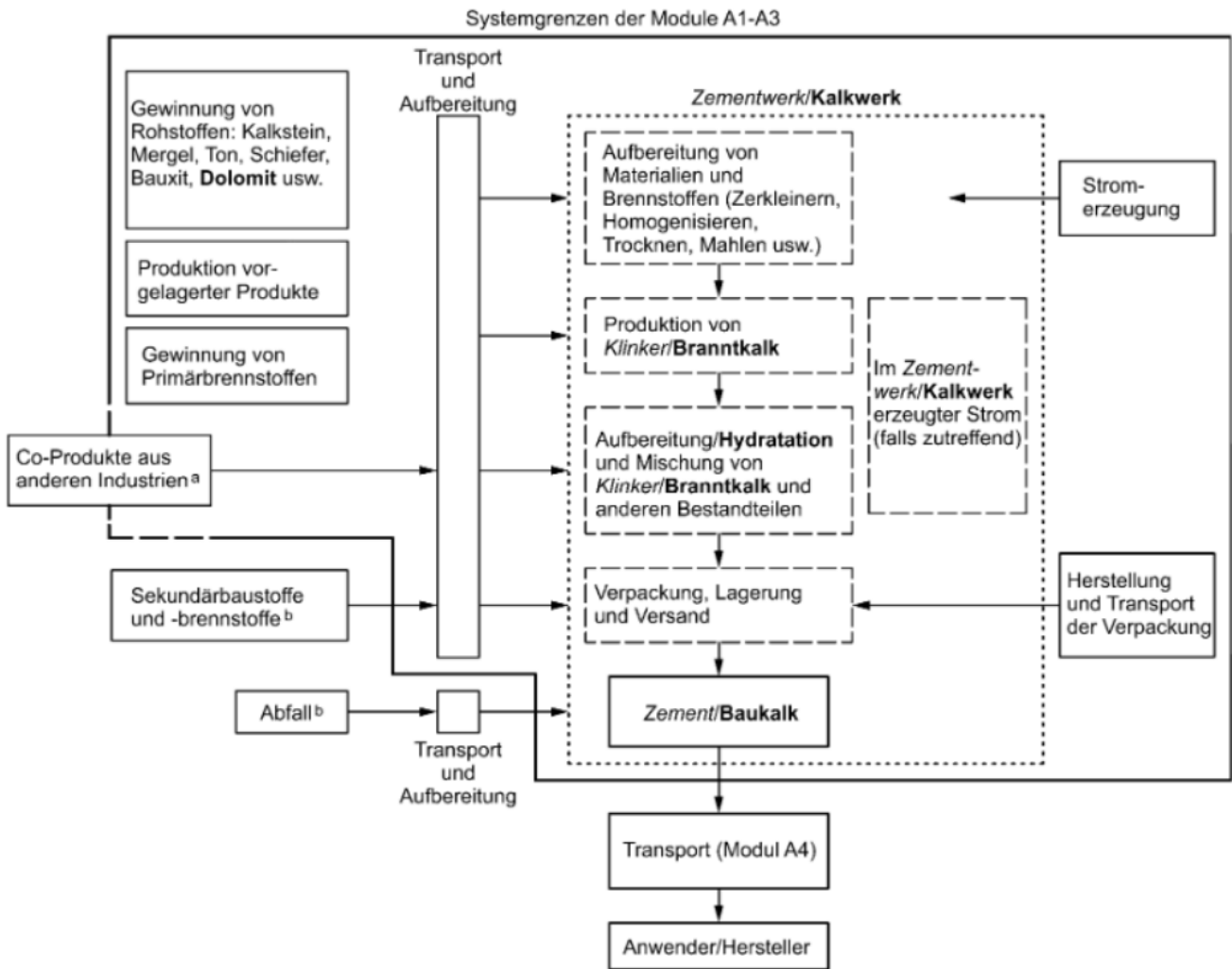
Abbildung 2: Systemgrenzen der Zementproduktion nach ÖNORM EN 16908 [20]
