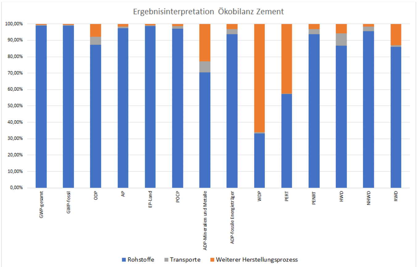
Abbildung 4: Dominanzanalyse Zementherstellung CEM II/A-S 52,5 R
