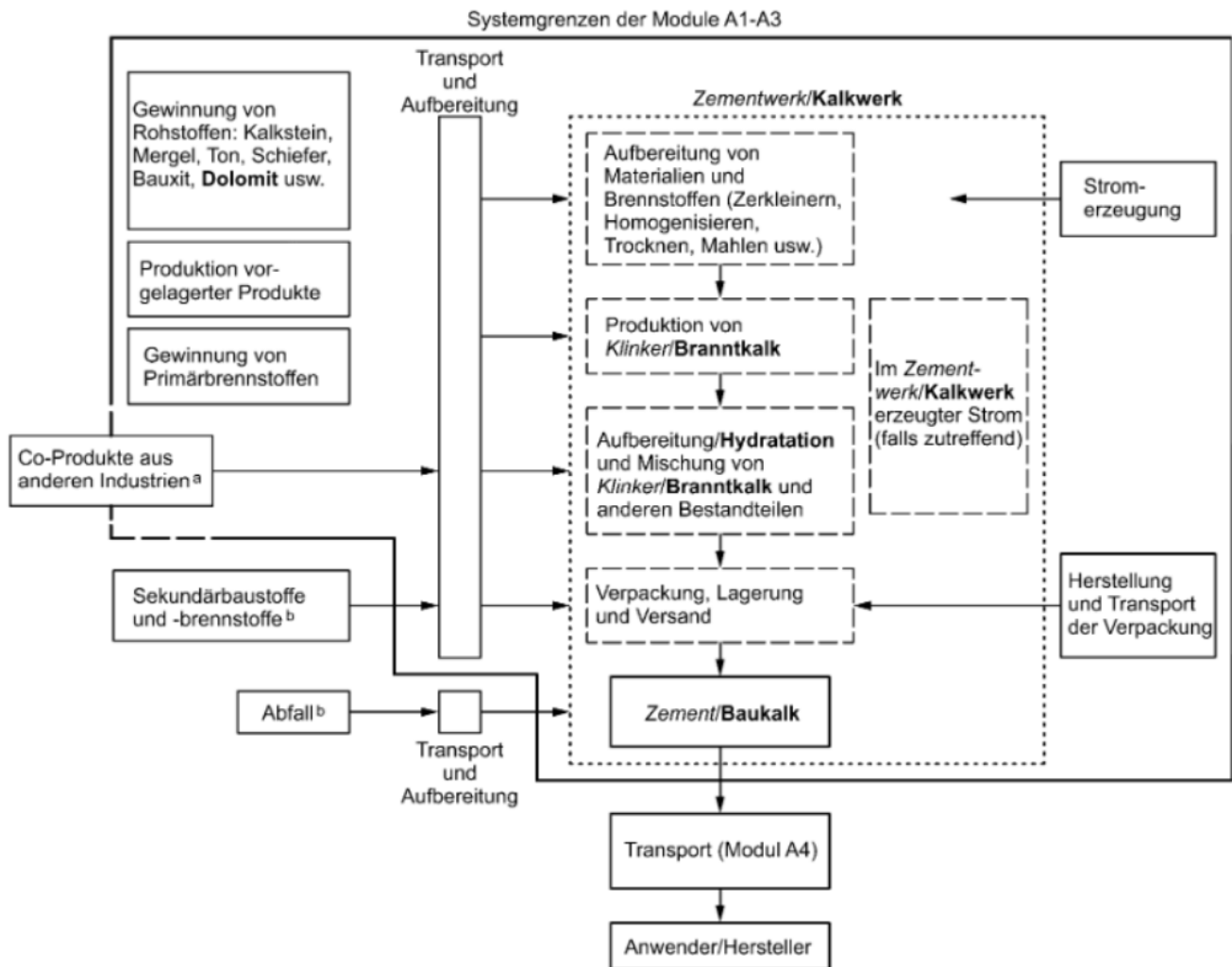
Abbildung 1: Systemgrenzen der Zementproduktion nach ÖNORM EN 16908 [6]
