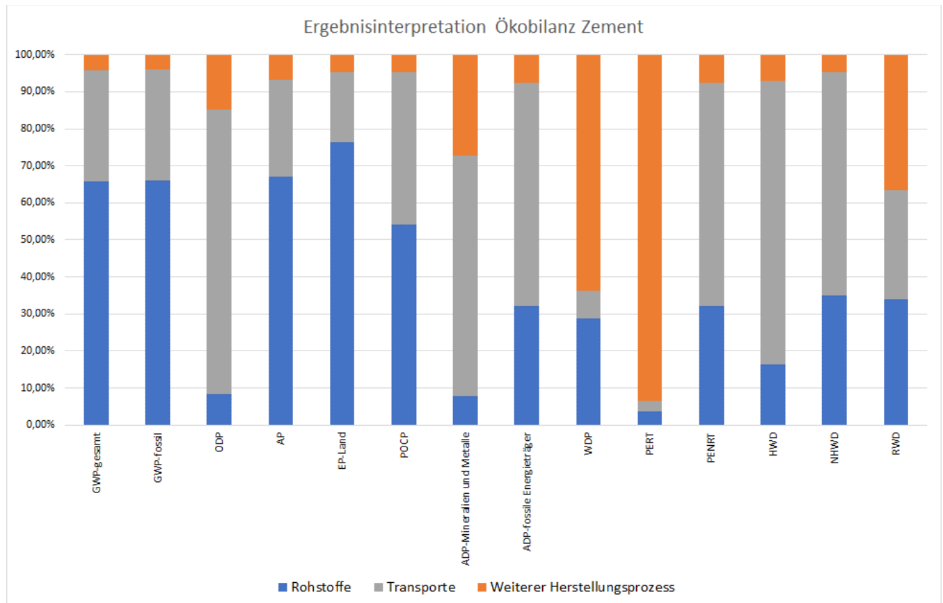
Abbildung 2: Dominanzanalyse Herstellung AHWZ LEUMIX
