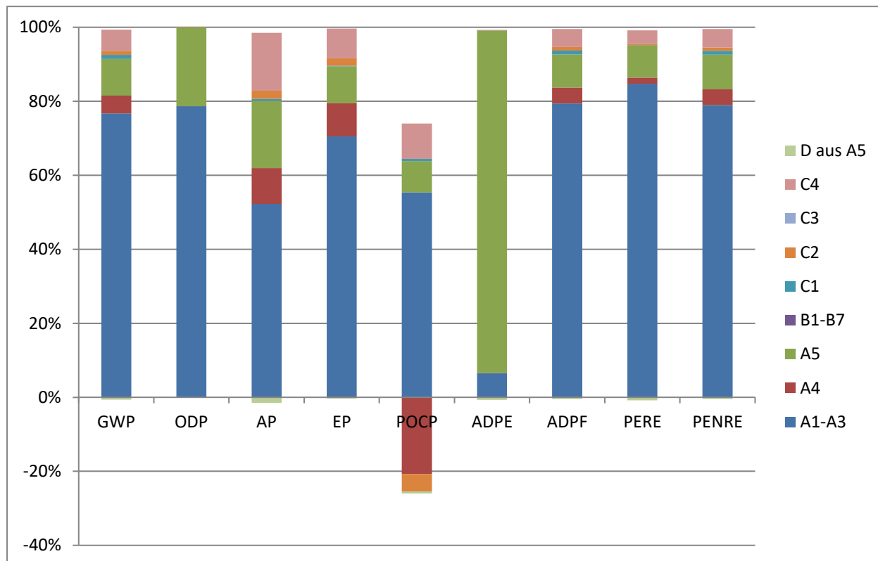
Abbildung 3: Durchschnittliche Anteile der Herstellungsphase A1-A3, des Auslieferungstransportes A4, des Einbaus A5, des Abbruchs, sowie des Entsorgungstransportes C2 und der Deponierung C4 der RIGIPS-Gipsplatten Duo`Tech RB, Duo`Tech RBI, Duo`Tech RF und Duo`Tech RFI mit einer Dicke von 25 mm.
