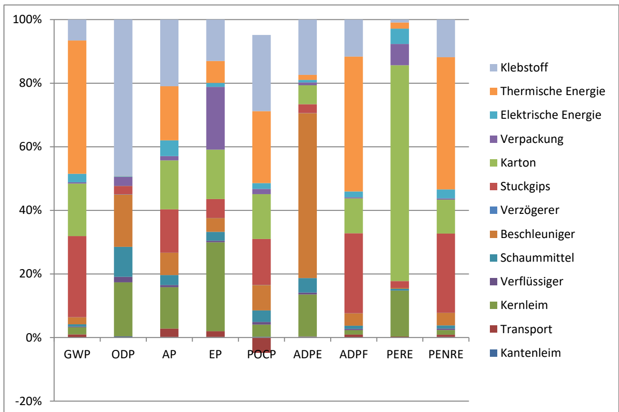
Abbildung 4: Durchschnittliche Anteile an der Herstellungsphase (A1-A3) für die RIGIPS-Gipsplatte Duo`Tech RB mit einer Dicke von 25 mm.
