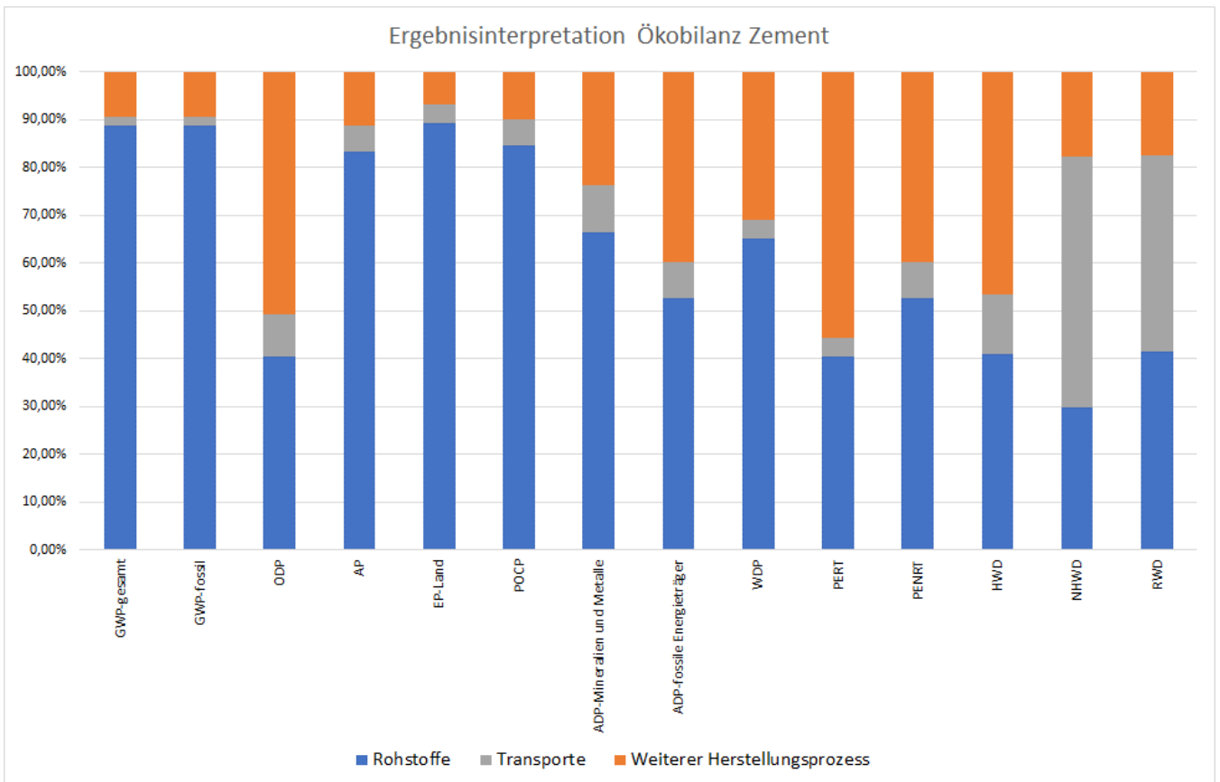
Abbildung 4: Dominanzanalyse Zementherstellung CEM III/B 32,5 N – SR
