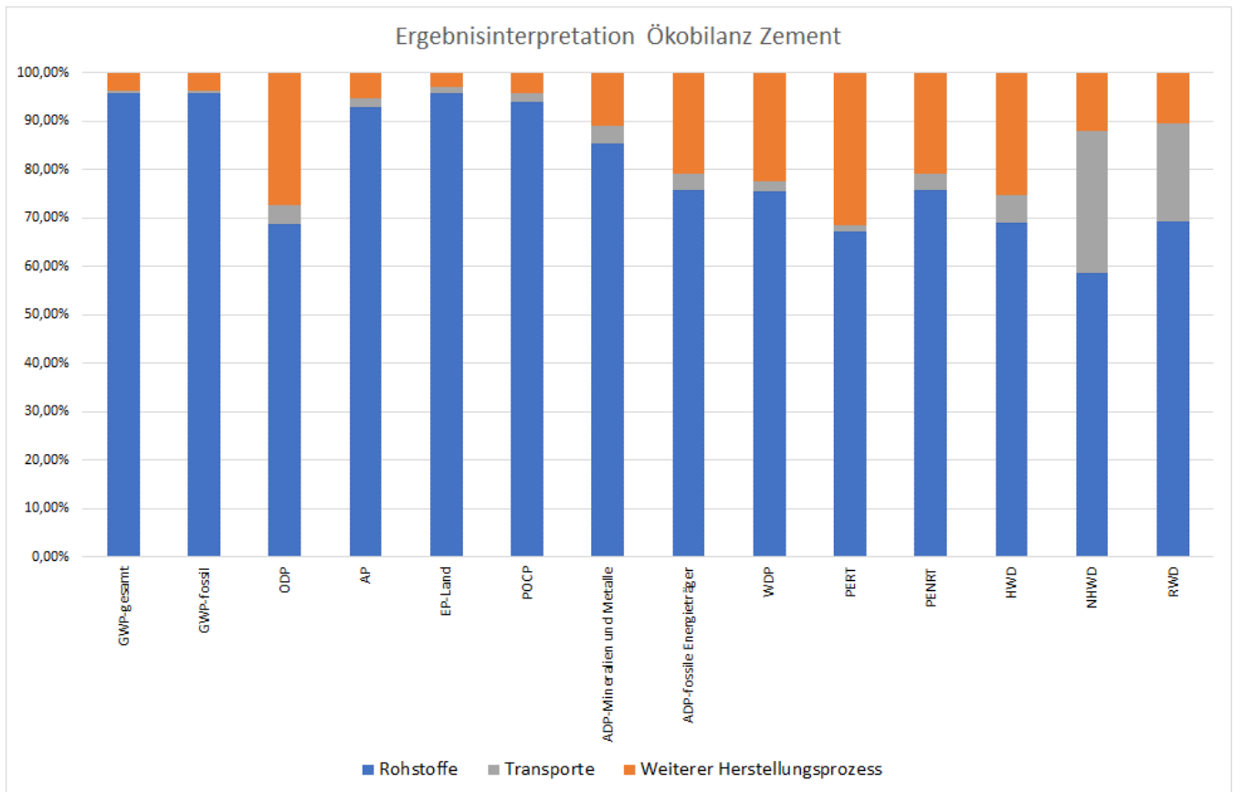
Abbildung 4: Dominanzanalyse Zementherstellung CEM II/B-S 42,5 N (DZ)
