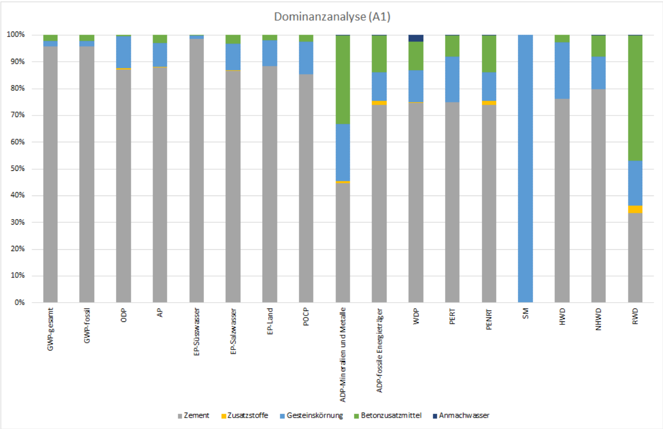
Abbildung 10: Dominanzanalyse Modul A1 Pflasterplatte
