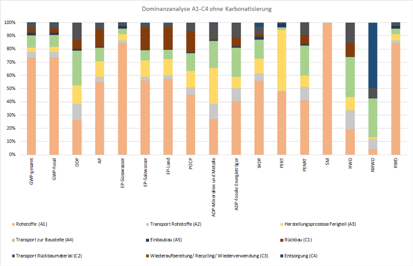
Abbildung 3: Dominanzanalyse Module A1-C4 Pflastersteine
