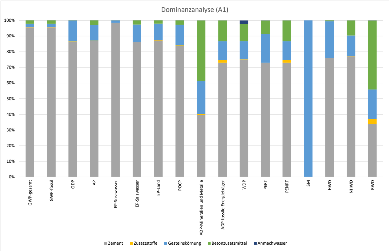
Abbildung 9: Dominanzanalyse Modul A1 Pflastersteine
