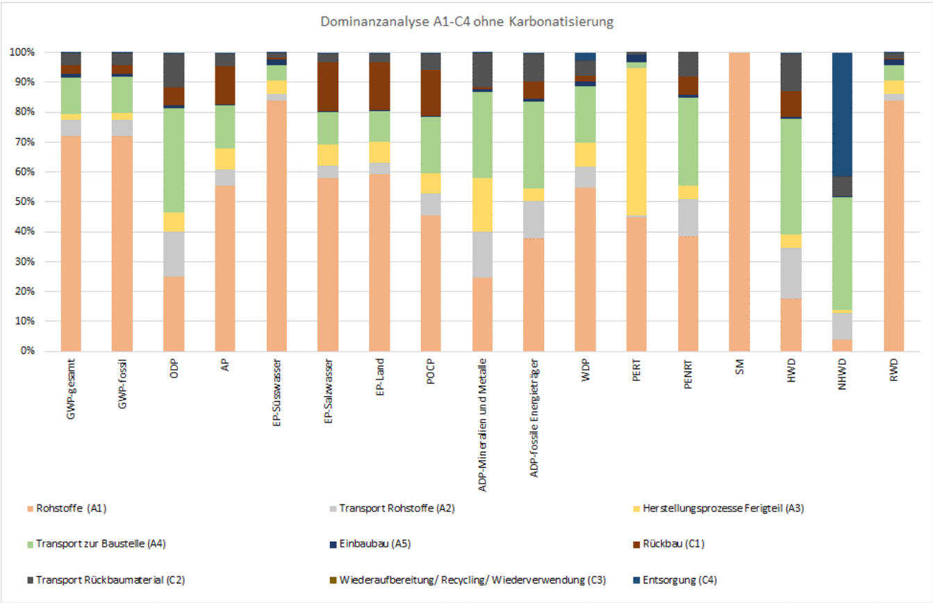
Abbildung 4: Dominanzanalyse Module A1-C4 Pflasterplatten
