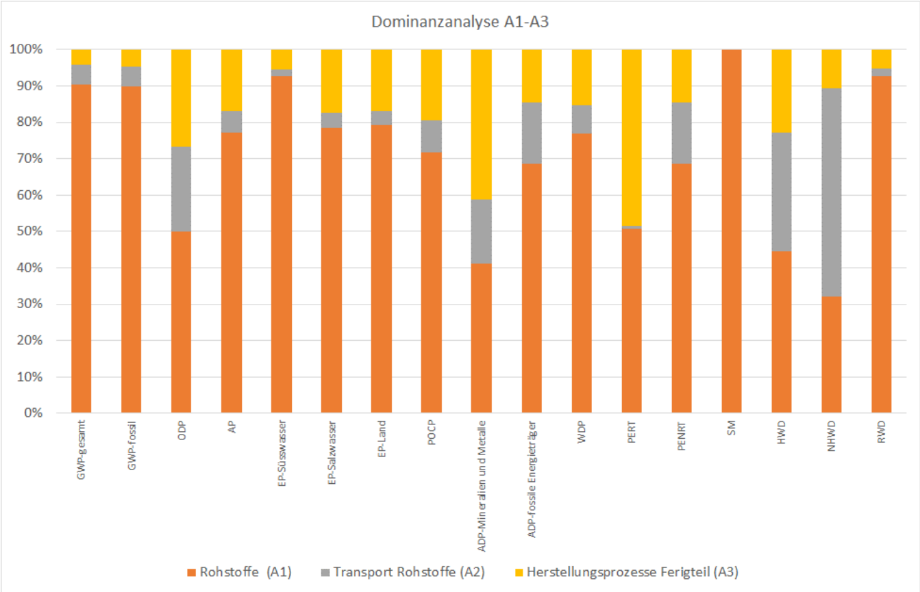
Abbildung 6: Dominanzanalyse Module A1-A3 Pflastersteine
