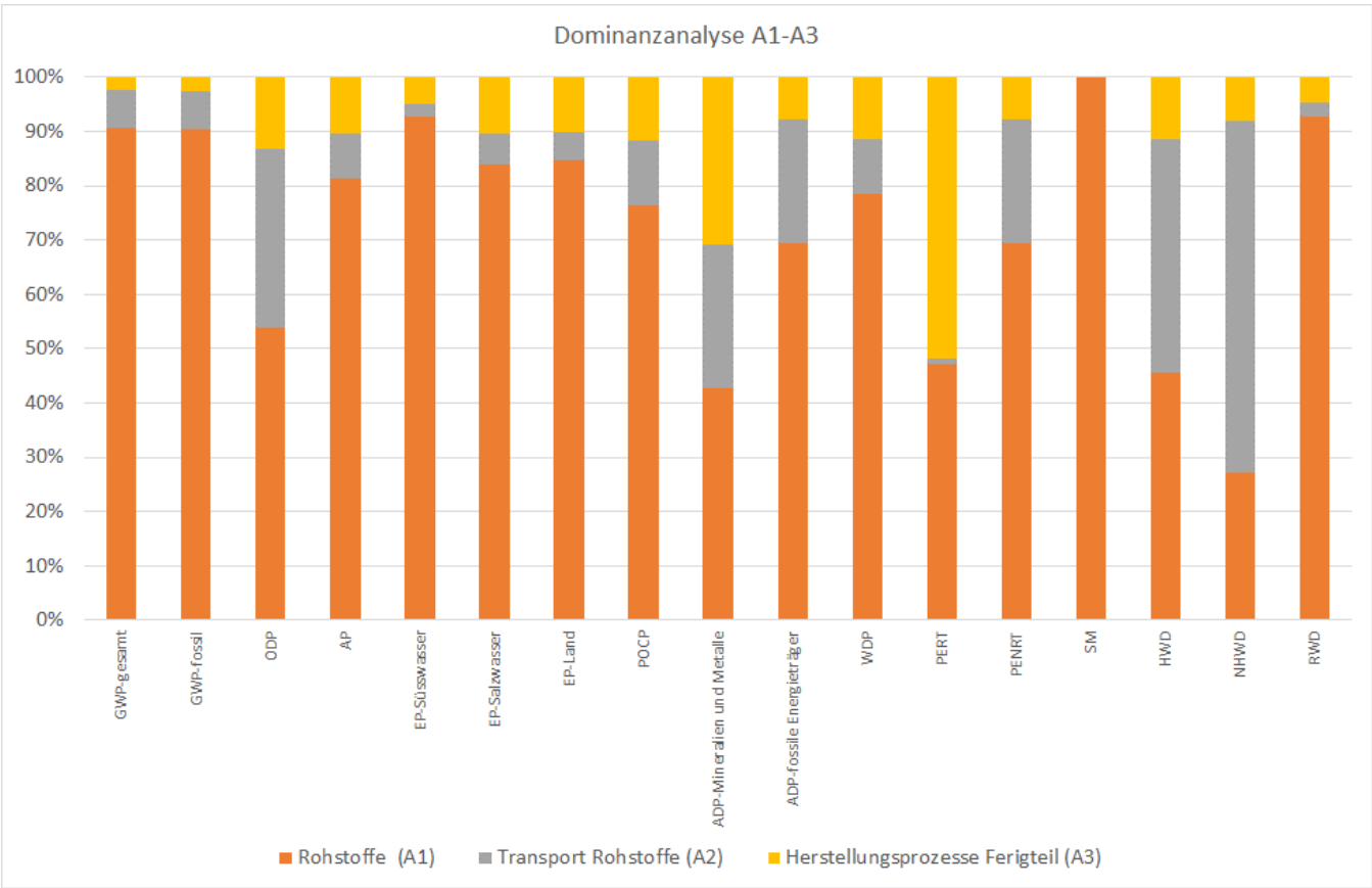
Abbildung 7: Dominanzanalyse Module A1-A3 Pflasterplatte
