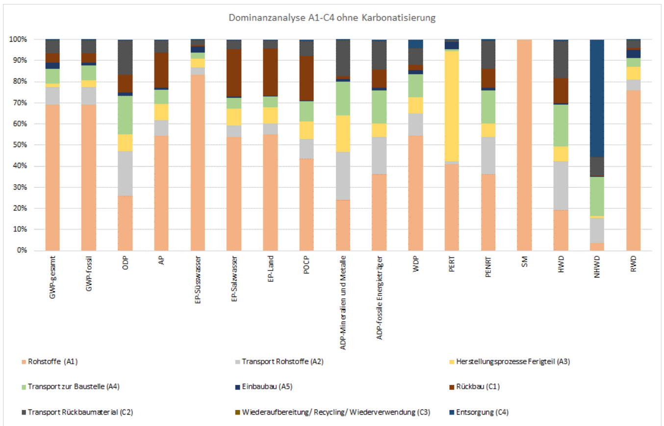
Abbildung 4: Dominanzanalyse Module A1-C4 Mauersteine/ Schalsteine
