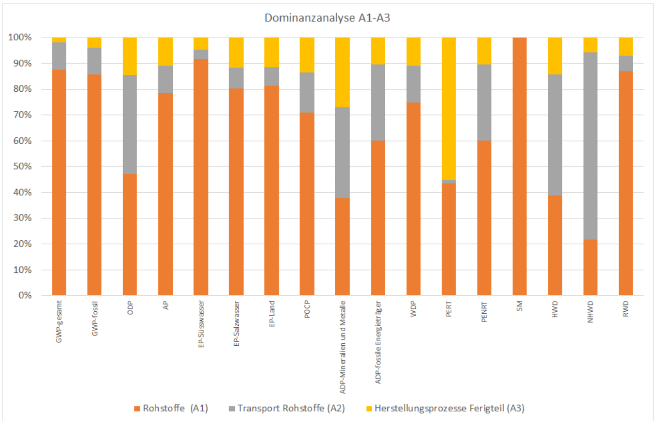
Abbildung 6: Dominanzanalyse Module A1-A3 Mauersteine/ Schalsteine
