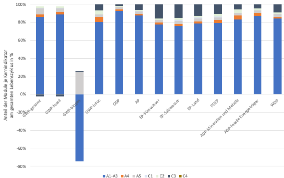
Abbildung 5: Beitrag der Lebenszyklusphasen zu den Kernindikatoren – (Szenario 1 – Recycling)
