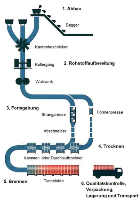
Abbildung 2: Schematische Darstellung des Produktionsablaufs (Initiative Ziegel, 2014)
