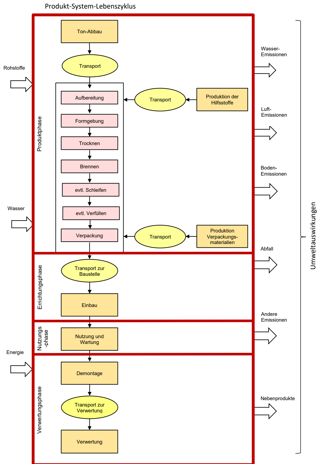
Abbildung 4: Flussdiagramm der Prozesse im Lebenszyklus, basierend auf (Initiative Ziegel 2014)
