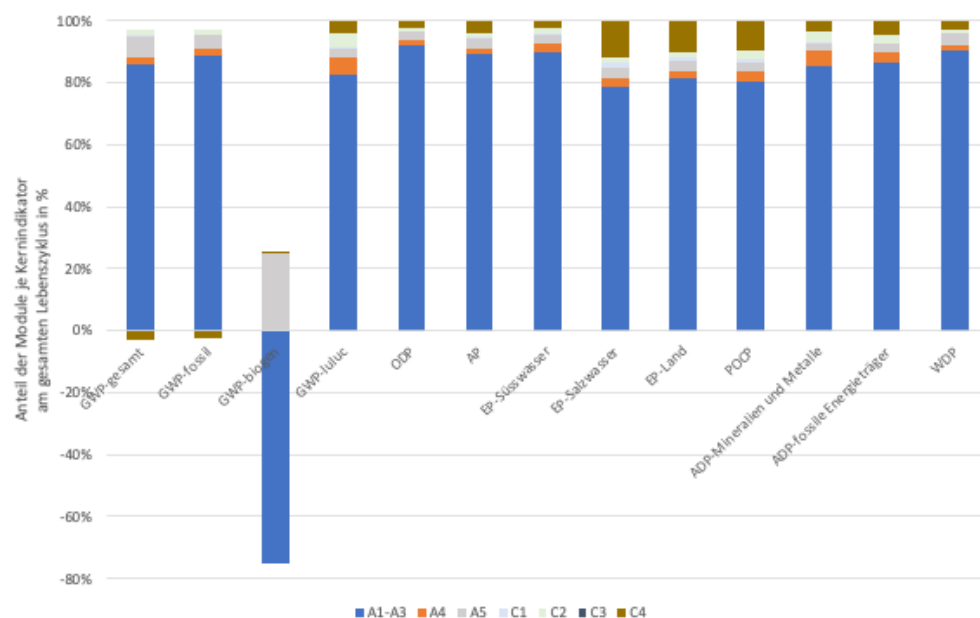
Abbildung 6: Beitrag der Lebenszyklusphasen zu den Kernindikatoren – (Szenario 2 – Deponierung)
