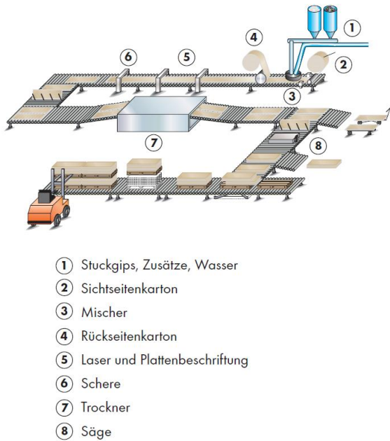
Abbildung 1: Beispiel eines Flussdiagramms Herstellungsprozesse
