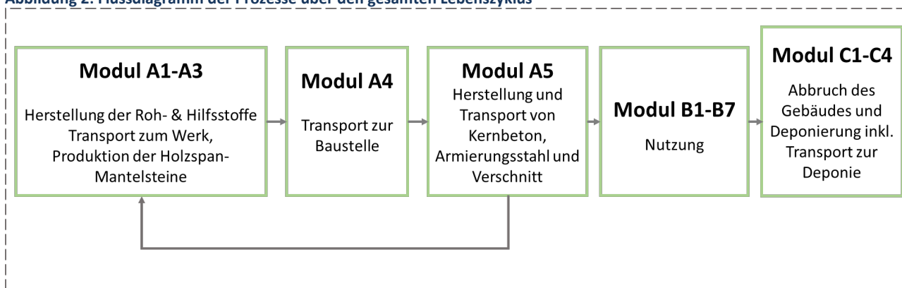
Abbildung 2: Flussdiagramm der Prozesse über den gesamten Lebenszyklus
