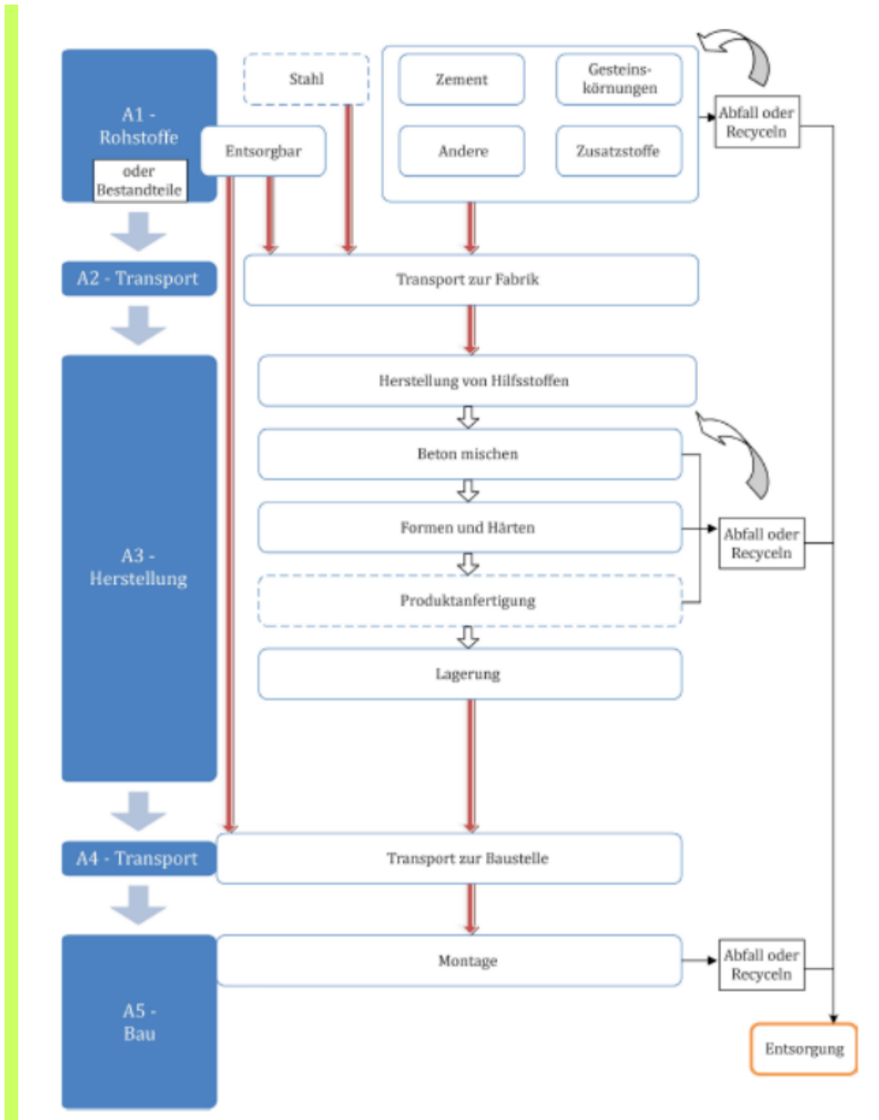
Abbildung 2: Systemgrenzen A1 – A5 für Betonfertigteilelemente
