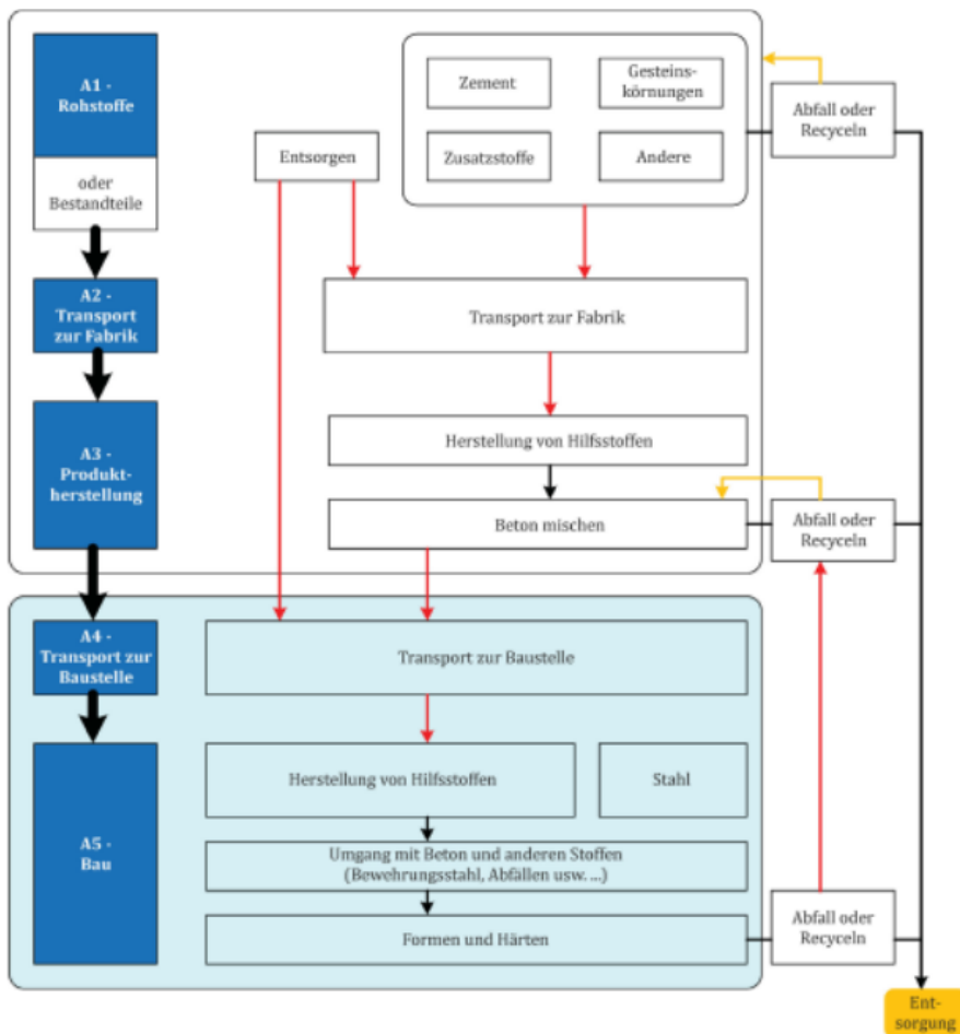
Abbildung 1: Systemgrenzen A1 – A5 für Transport- und Baustellenbeton
