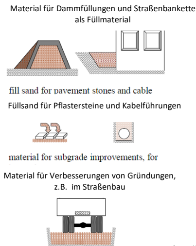
Abbildung 4: Beispiele für die Anwendung von Ziegelsplitt in ungebundenen Systemen
